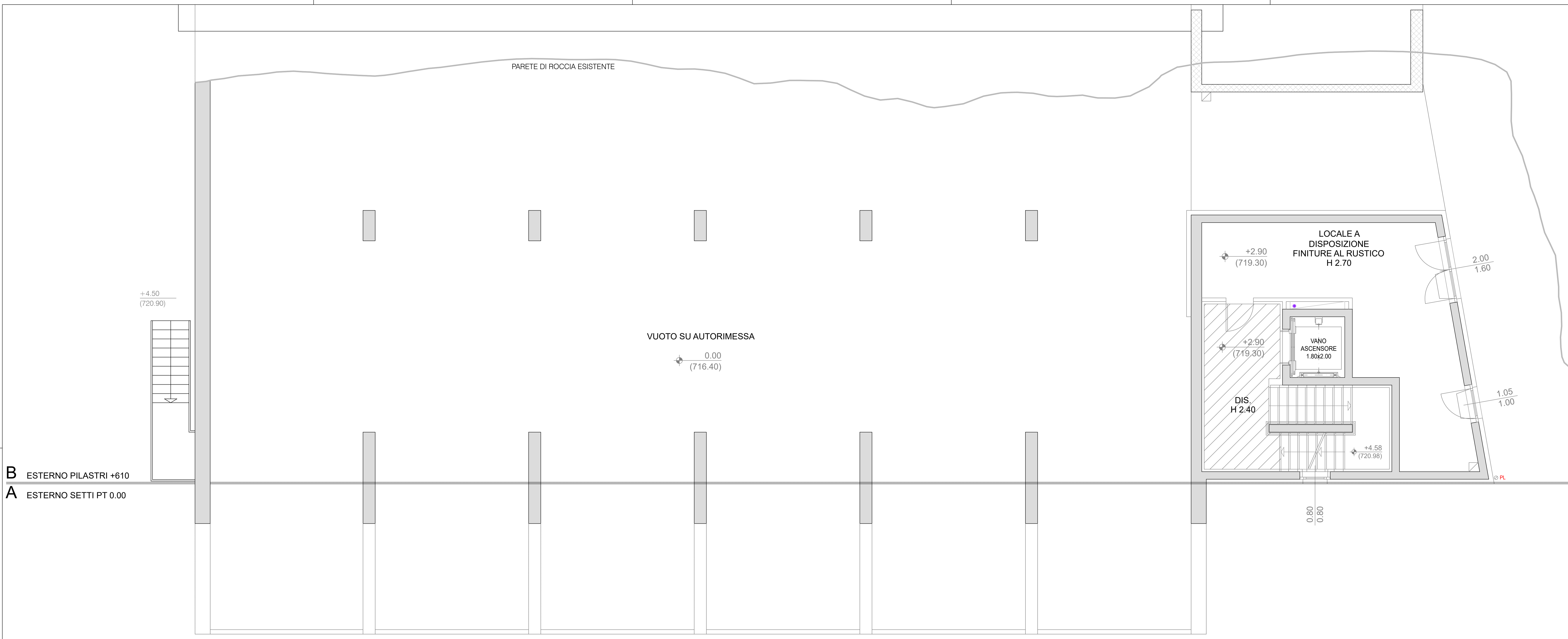
PIANTA PIANO +2,90
